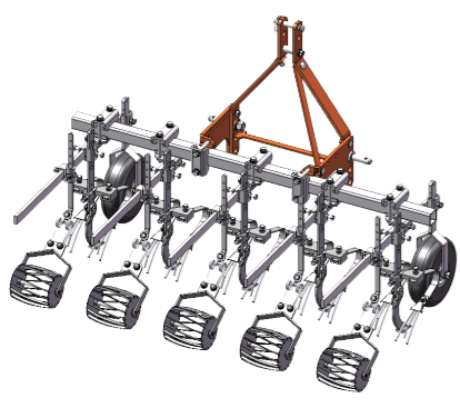
●新玉除草カルチ A 4畦 (レーキ無・玉ねぎクラッシャー付) 型式：H018-4BHA 玉ねぎの中耕に最適。
