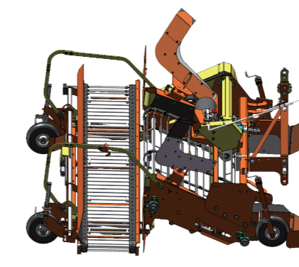
●デガー (ロッドタイプ・タイヤ手動) 型式：H040-1EHA 玉ねぎの集積、堀取に最適。
