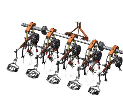
●ハイテクカルチ5畦 (碎土輪・碎土クラッシャー・ウルトラQ付) 型式：H003-5JHA ビート・豆等の中耕除草に最適。
