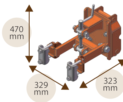
三菱用ヒッチ (MPR65用)
