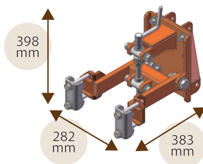
クボタ用ヒッチ (SPU用)
